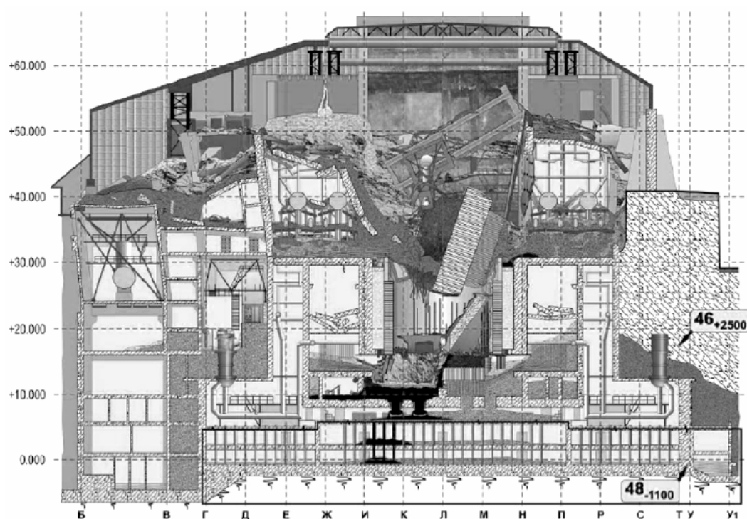
Figura 3. Sezione del “sarcofago” con lo stato del reattore poco dopo dopo l’esplosione.
